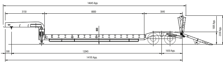
■ 外観図面
