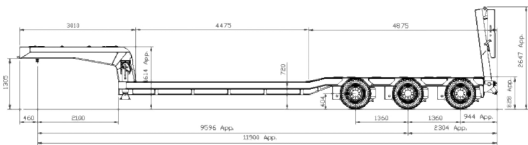
■ 外観図面
