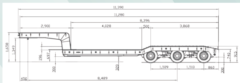
■ 外観図面
