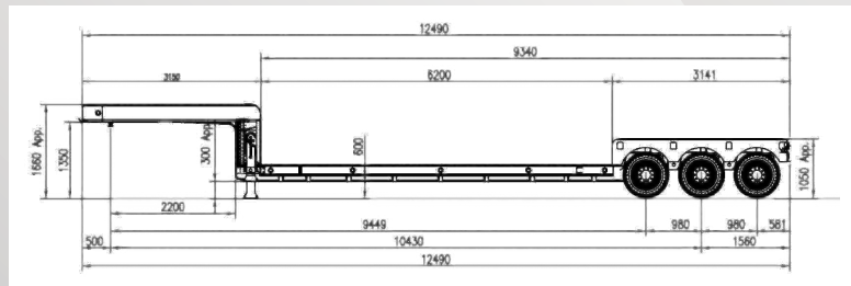
■ 外観図面
