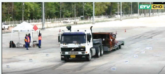
■ 制動試験積載(乾燥路)
